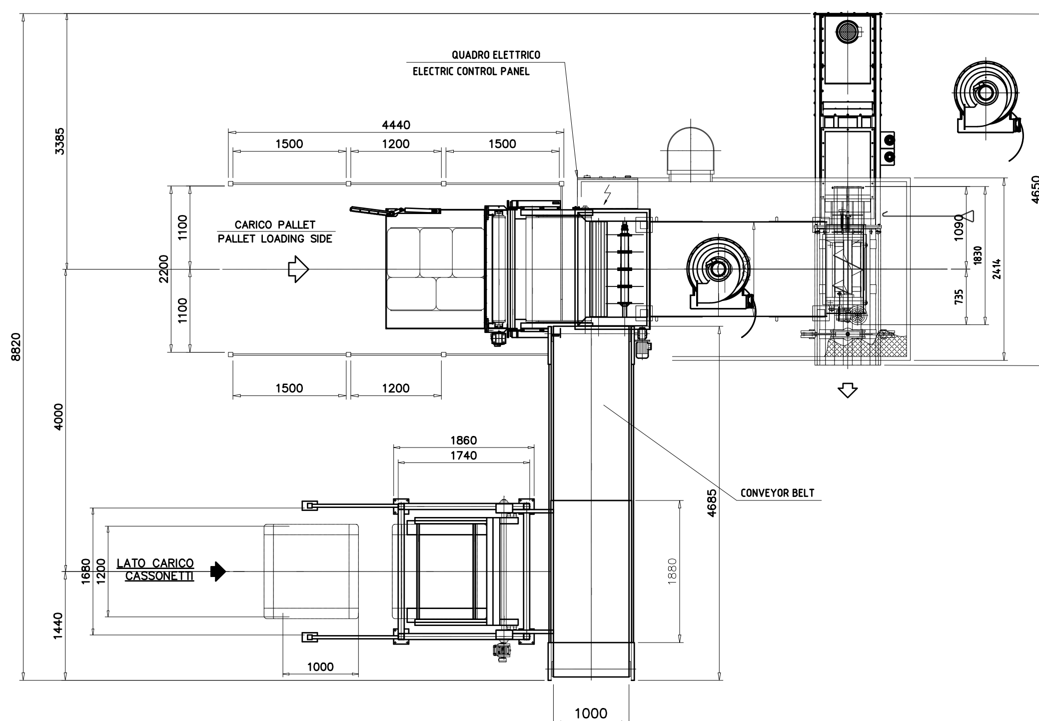
VISTA CON RIBALTATORE SKIP VIEW WITH TIPPER SKIP
